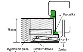
PROFIL SKRZYDŁA
