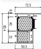
Rysunek techniczny
