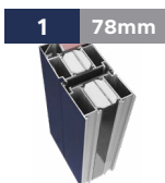
1 78mm Ciepła ościeżnica z poliamidową przekładką termoizolacyjną
