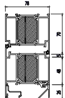
Rysunek techniczny
