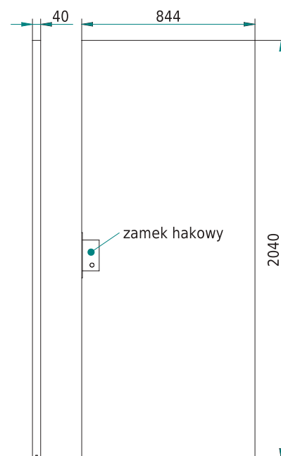
skrzydło przesuwne
