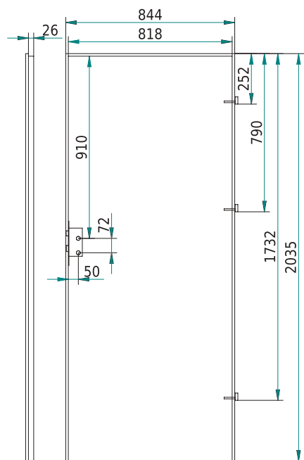
skrzydło przylgowe
