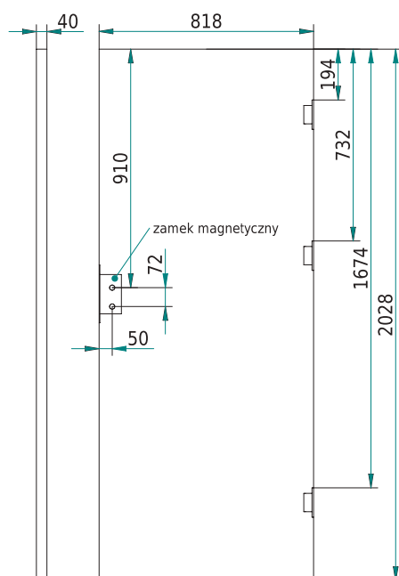
skrzydło bezprzylgowe
